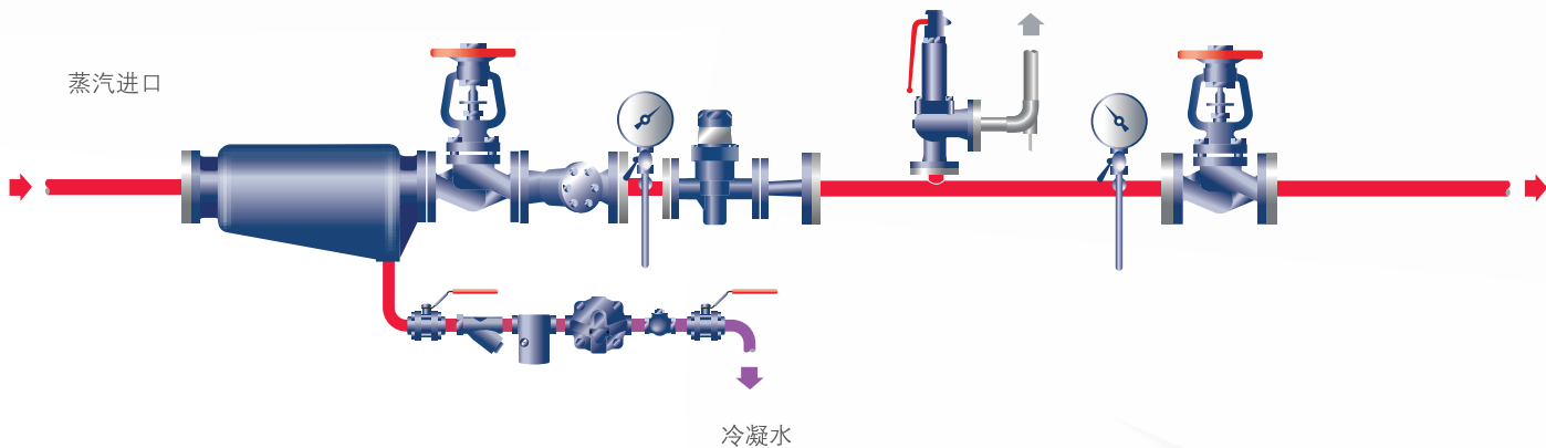
典型的减压站布置图
